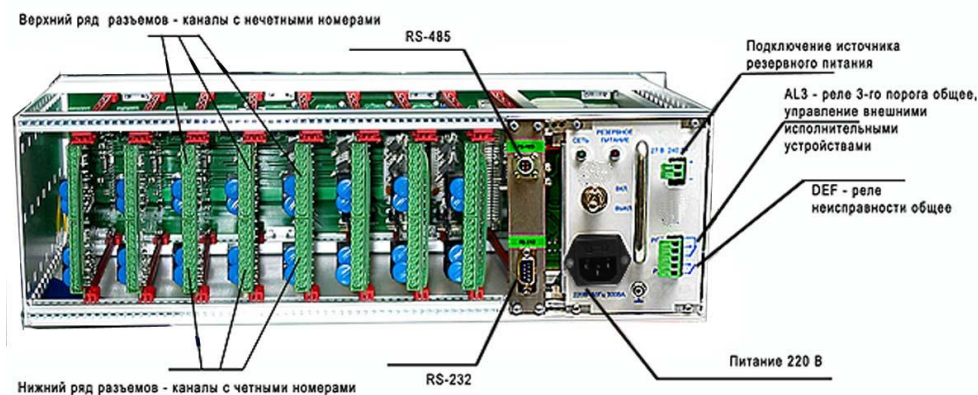
Рисунок А.1 – Общий вид терминала
