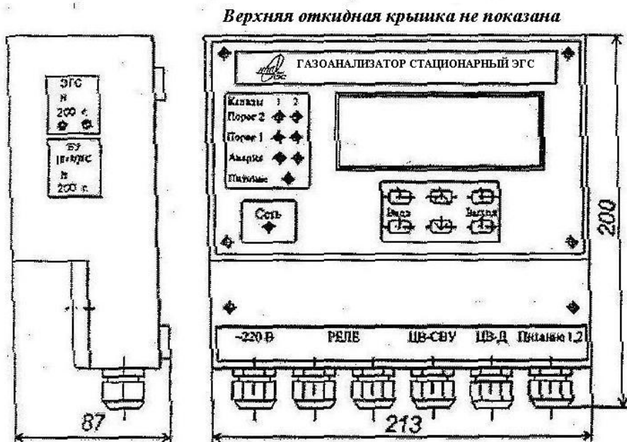
Рисунок А3 – БУ уменьшенных габаритов
